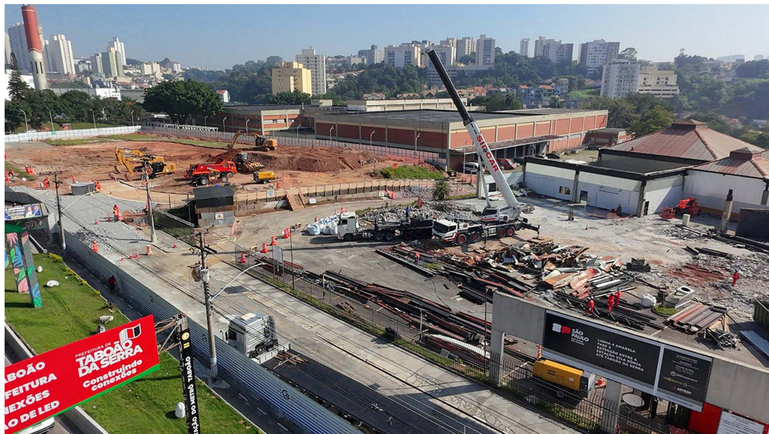
Início das escavações marca avanço da construção da estação Taboão da Serra da Linha 4-Amarela do Metrô
